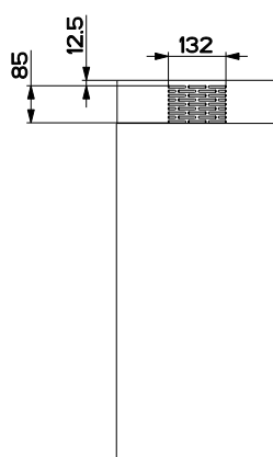
VUE ARRIÈRE
